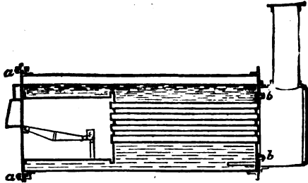
Фиг. 5. Котель Л. системы Вольфа.
